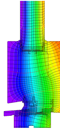
Isothermengrafik
