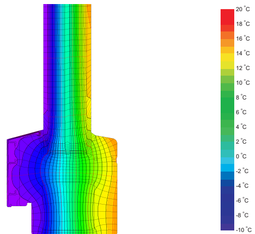
Isothermengrafik
