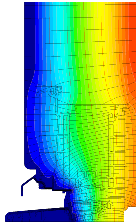
Isothermengrafik
