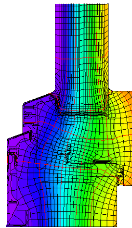
Isothermengrafik
