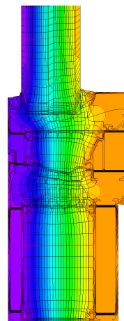
Isothermengrafik
