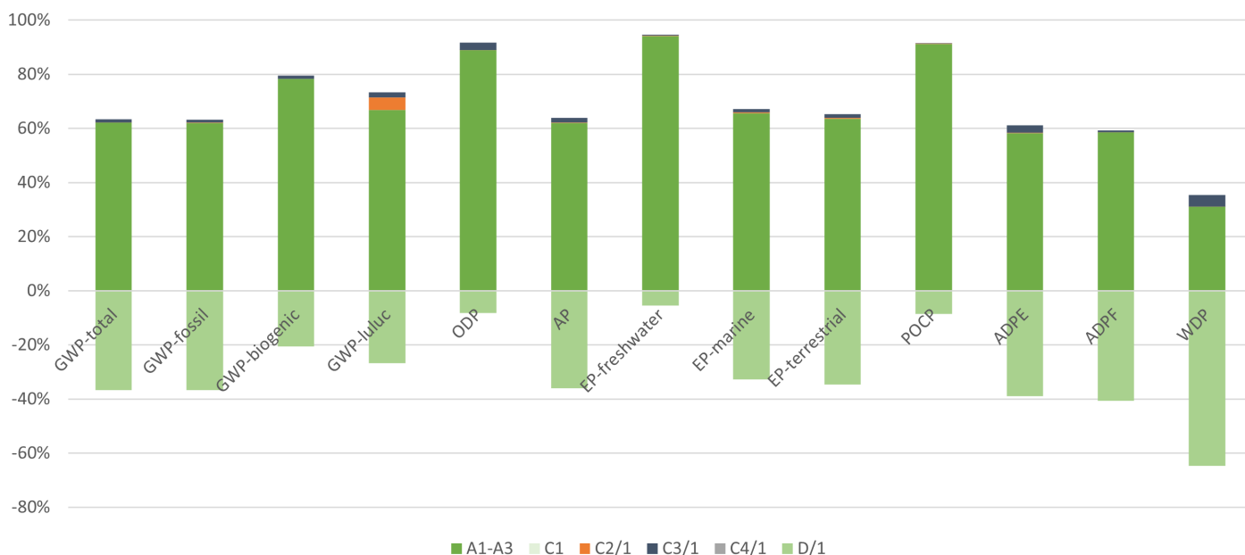
Relative Beiträge der verschiedenen Lebenszyklusphasen der blaugelb Triotherm+ Profile – klassisch (100% stoffliches Recycling)
