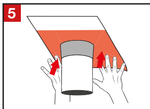
Unteren Teil des Klebekragens fest andrücken.
