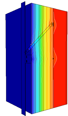
Isothermenbild Festpunkt
