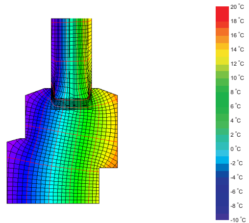
Isothermengrafik
