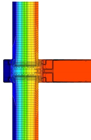
Isothermengrafik
