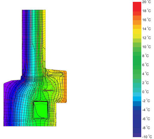
Isotherme
