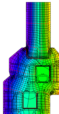
Isothermengrafik
