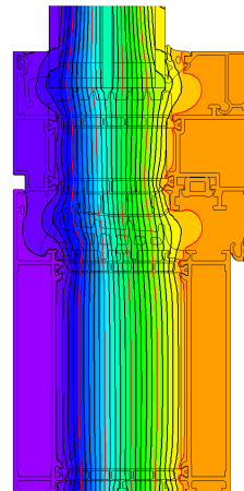
Isothermengrafik
