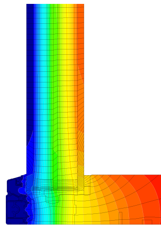
Isothermengrafik
