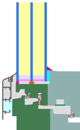
Berechnungsmodell
