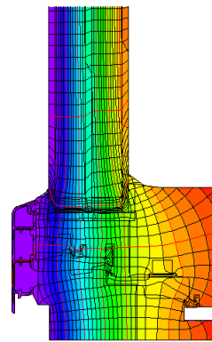
Isothermengrafik
