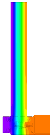
Isothermengrafik
