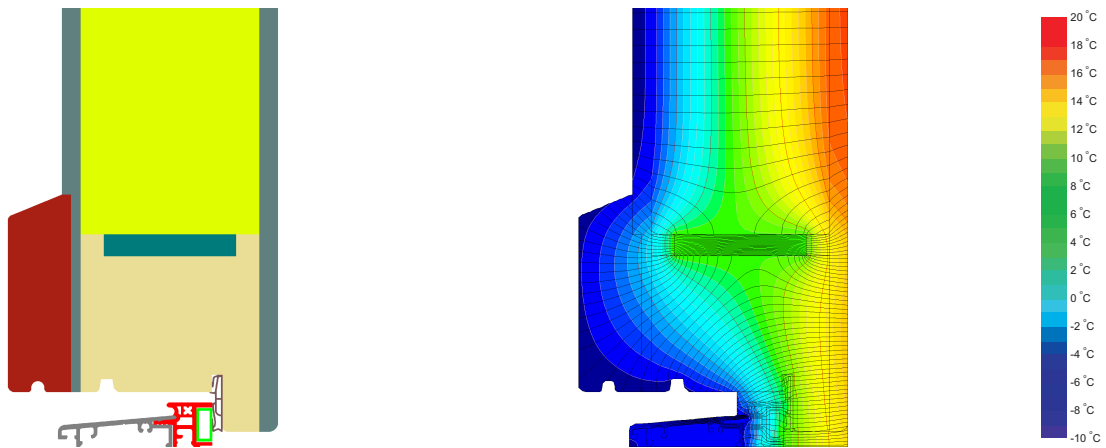
Berechnungsmodell
