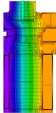
Isothermengrafik
