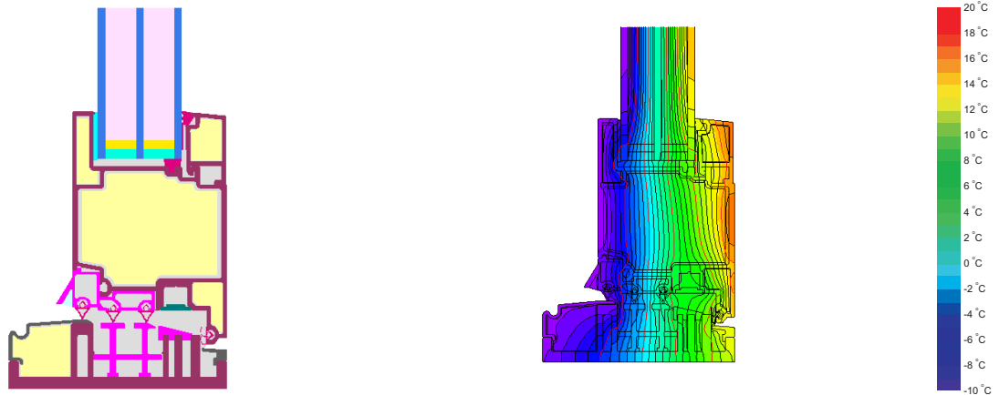
Berechnungsmodell
