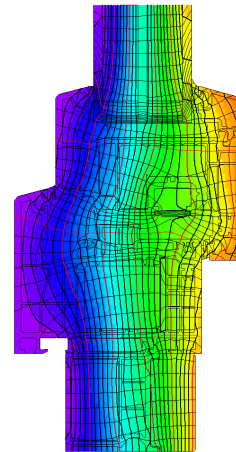
Isothermengrafik
