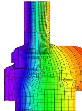
Isothermengrafik
