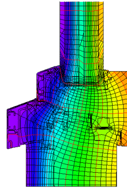
Isothermengrafik
