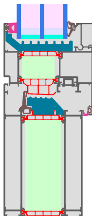
Berechnungsmodell
