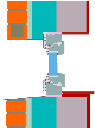
Zweischaliges Mauerwerk
