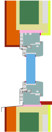
Holzleichtbau (öffnenbar)
