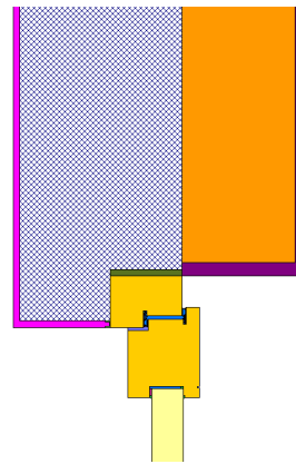
Schwelle Eingangstür
