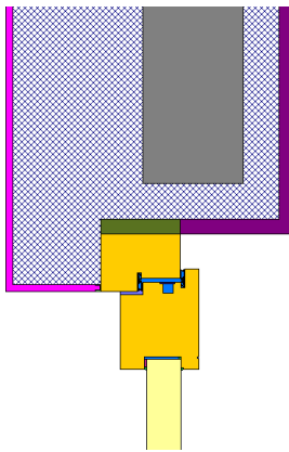
Holzleichtbau (öffnbar)
