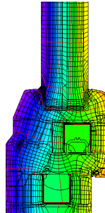
Isothermengrafik
