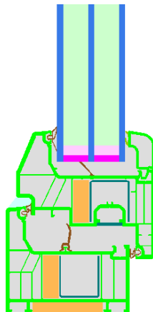
Berechnungsmodell
