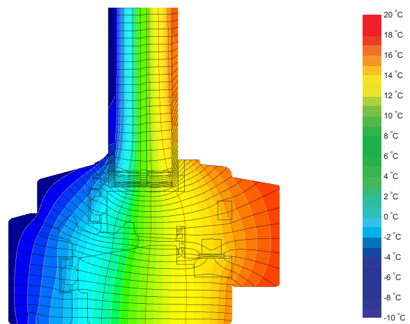
Isothermengrafik
