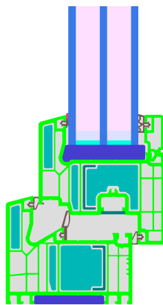
Berechnungsmodell
