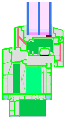
Berechnungsmodell
