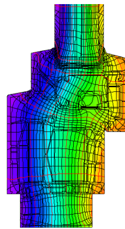
Isothermengrafik
