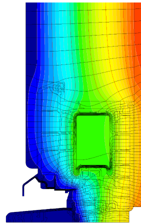
Isothermengrafik
