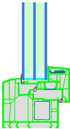
Berechnungsmodell
