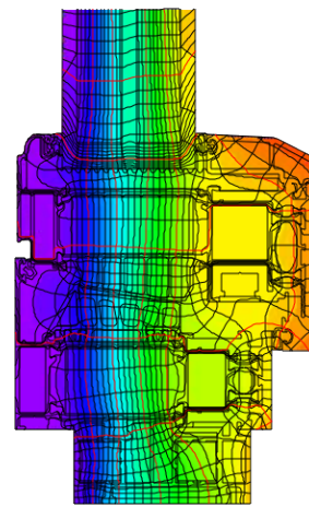
Isothermengrafik
