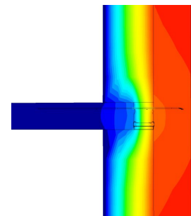
Isothermenbild des XT Typ K-WO-M2-V1
