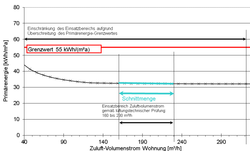
Abbildung 2: Einsatzbereich des Gerätes bezüglich des Zuluftvolumenstroms.
