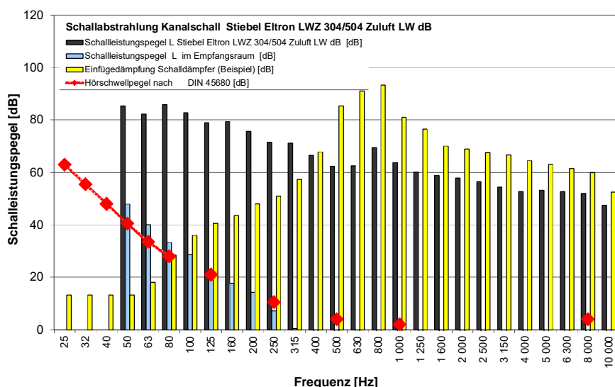
Abbildung 1: Schallabstrahlung Zuluftkanal
