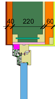
Wärmedämmverbundsystem (WDVS) Schwelle Geschossdecke (öffnbar)
