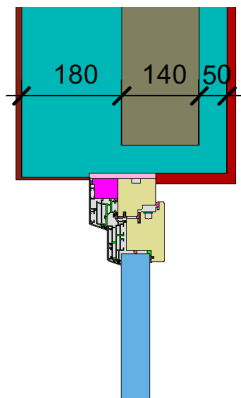
Wärmedämmverbundsystem (WDVS) oben (öffnbar)
