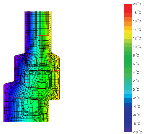
Isotermas
