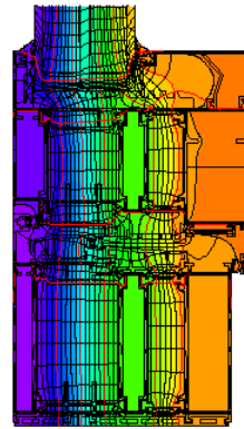
Isothermengrafik
