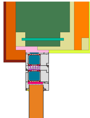
Wärmedämmverbundsystem (WDVS) (öffnbar)
