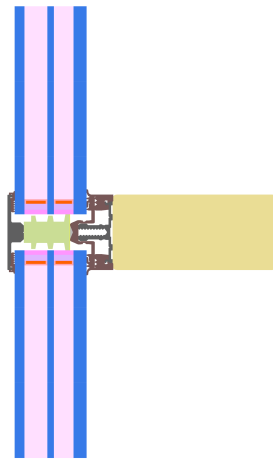
Berechnungsmodell
